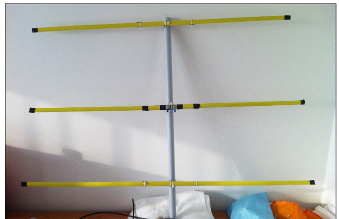
Antennitöötoa tulemus: igati kasutatav 2m yagi!
