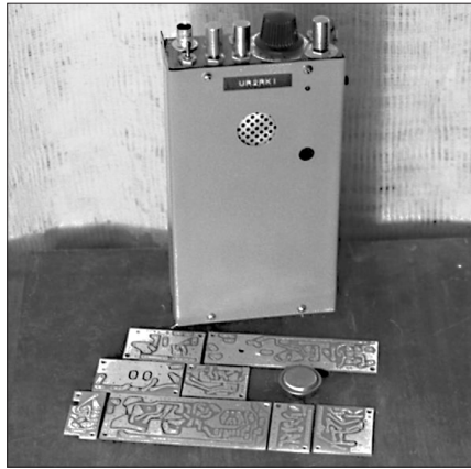
UR2RKI poolt 1986.a. valmistatud 2m FM-käsijaam
