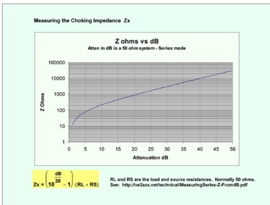
Pilt 4. NanoVNA-ga mõõtmisel saadud impedantsi ja sumbuvuse seos
